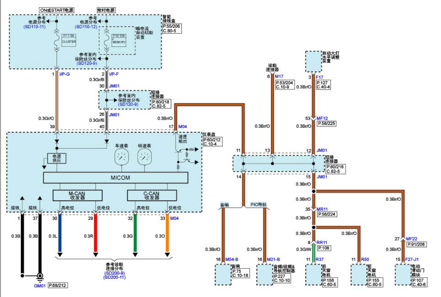
车速系统(1)
